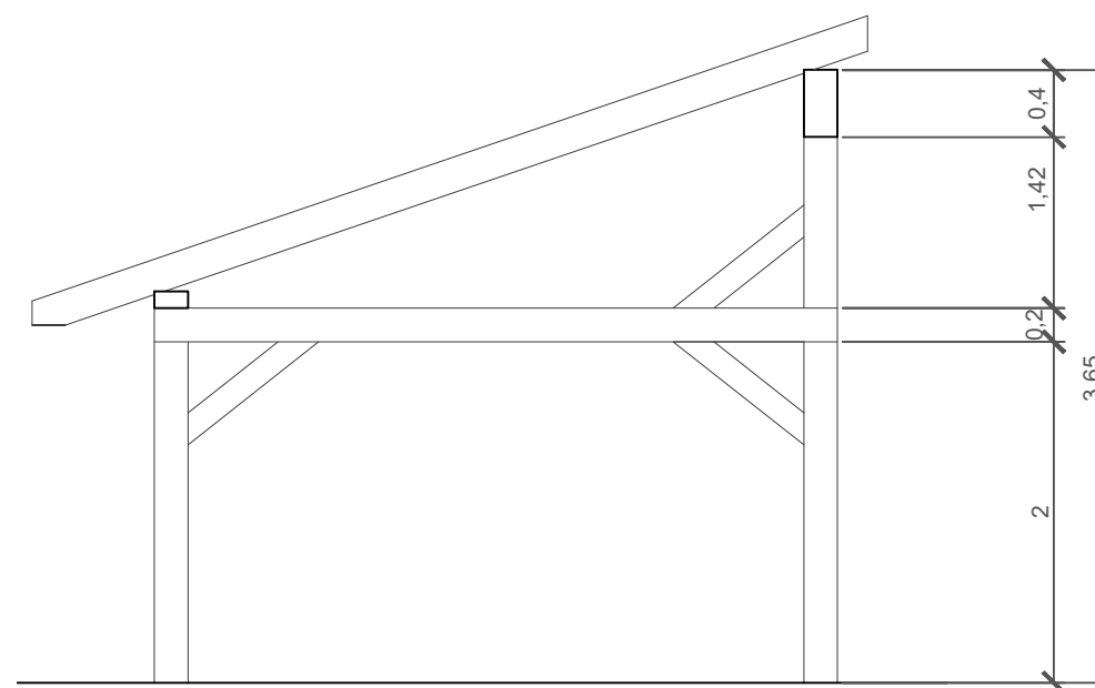
ALÇADO 1.50
